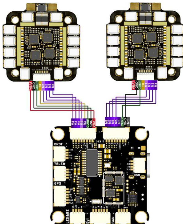
Příklad propojení s řídicí jednotkou FlyingRC H7D podle podkladů výrobce
