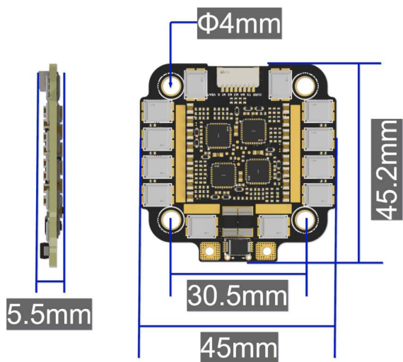
Rozměry regulátoru
