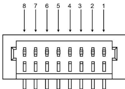
Číslování pinů konektoru SH1.0 8P
