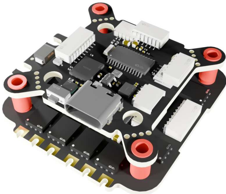
Sestava řídicí jednotky F4D MK1 a 4v1 regulátoru otáček 45 A
