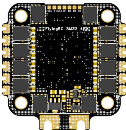
Spodní strana regulátoru s ploškami motorů M1 až M4
