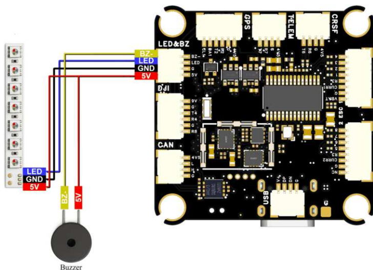
Připojení LED pásky a bzučáku podle podkladů výrobce
