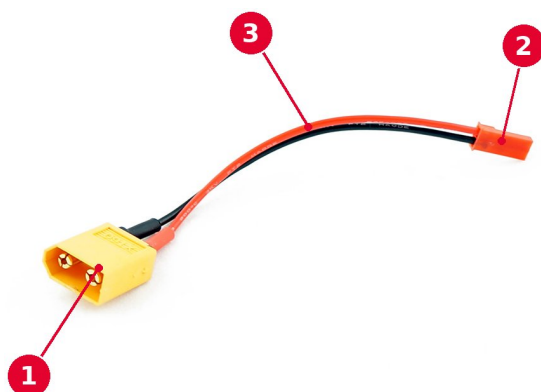
① konektor XT60 (samec) · ② konektor JST (samice) · ③ propojovací vodiče – červený (+), černý (–)
